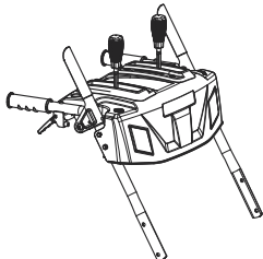
Верхняя рукоятка в сборе x 1
